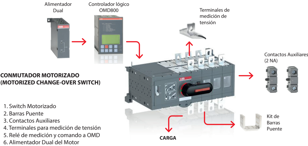
SWITCHES MOTORIZADOS
